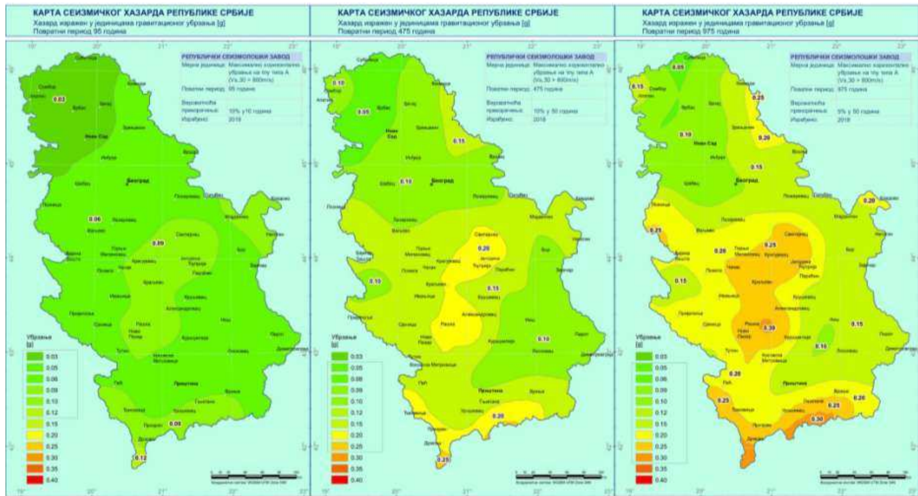
Слика: Карта максималног гравитационог убрзања
