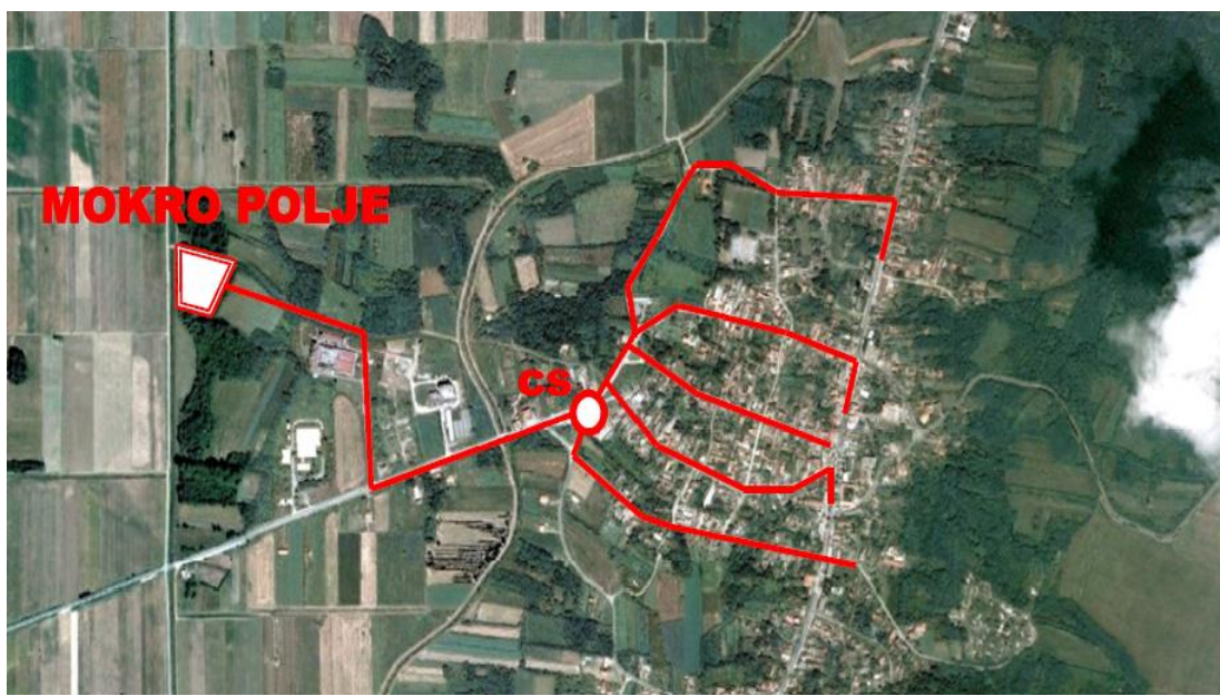
Постојећа канализациона мрежа и Мокро поље у насељу Жабари;
