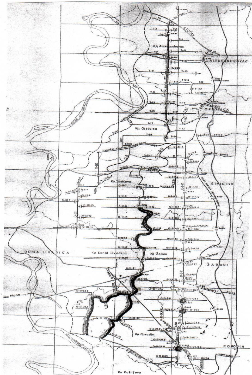
Слика 27. Каналска мрежа на територији општине Жабари;
